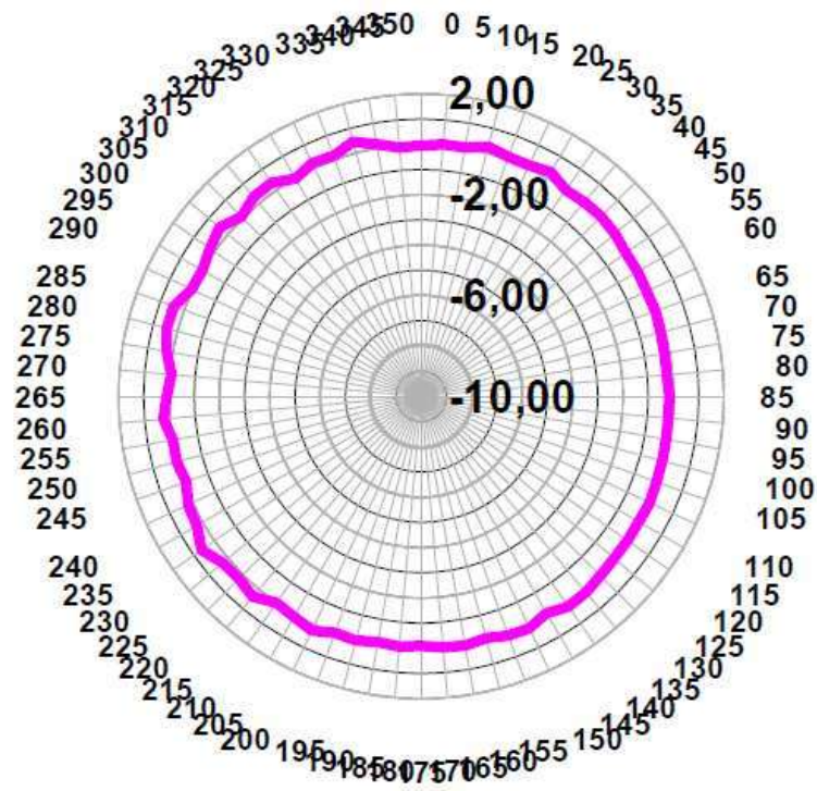
Freq. 900 MHz H-plane (dBi) V-pol
